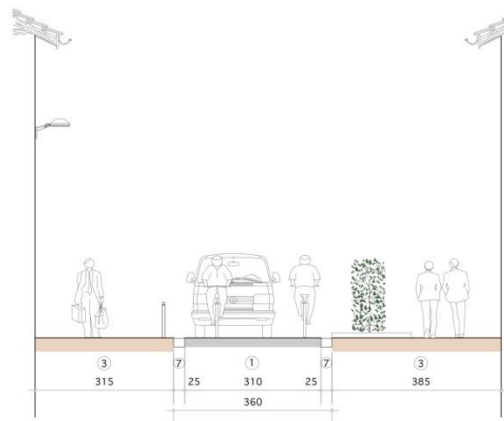
Coupe/Snede BB
