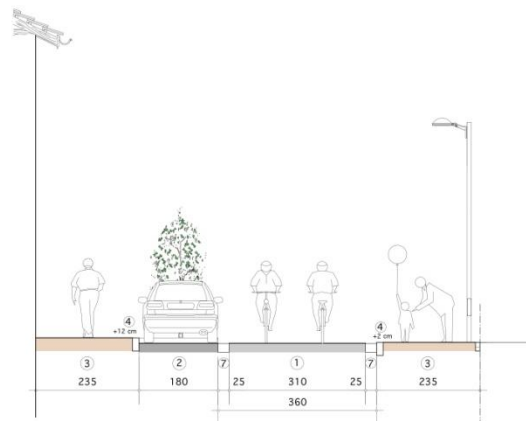
Coupe/Snede AA
