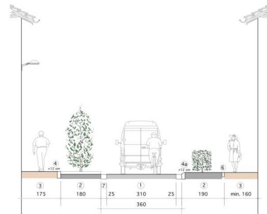
Coupe/Snede CC
